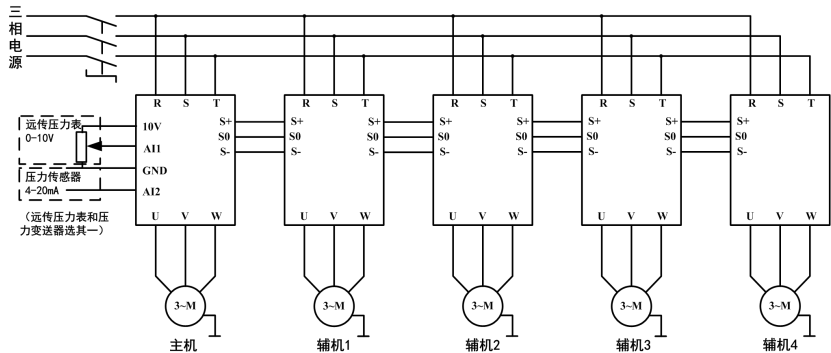
图3-1-4 联机接线图
