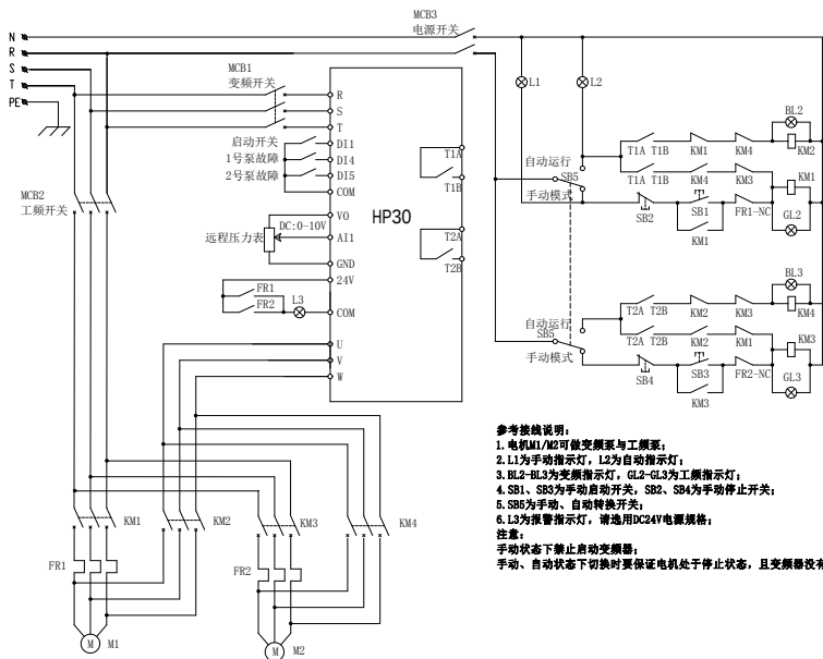
0.75-7.5kW一拖二电路图
