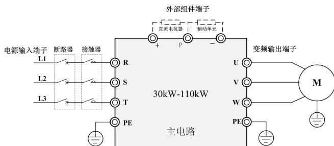
图 2-5-2 30kW-400kW 主端子示意图
