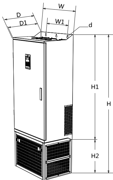
图 2-3-3 132kW-400kW 外形尺寸示意图
