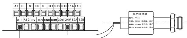
图 2-7-3 0.75-7.5kW 两线制压力变送器接线图
