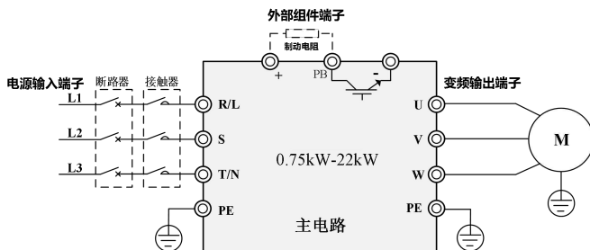
图 2-5-1 0.75kW-22kW 主端子示意图
