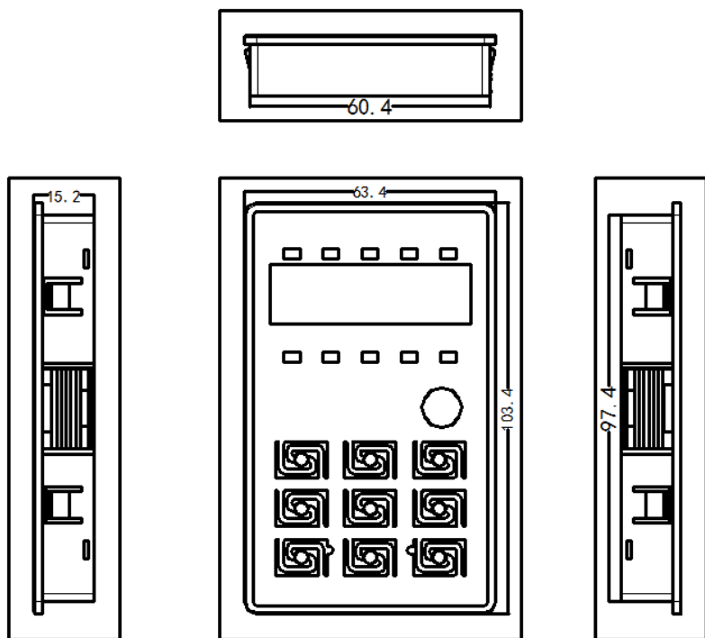
图 2-4-2 0.75kW—400kW 键盘尺寸图
