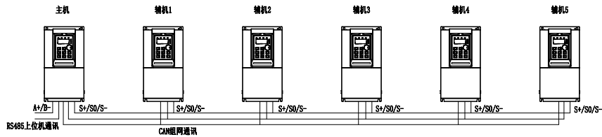
图 3-1-2 联机示意图
