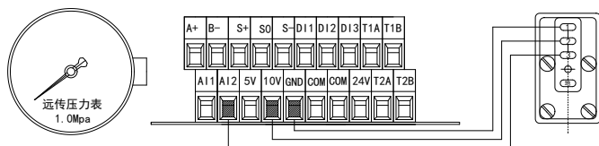
图 2-7-1 0.75-7.5kW 远传压力表接线图
