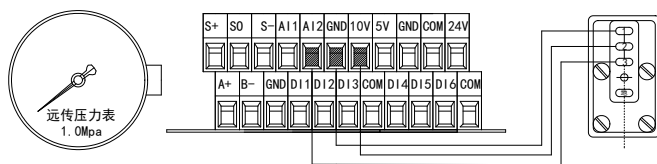
图 2-7-2 11-400kW 远传压力表接线图
