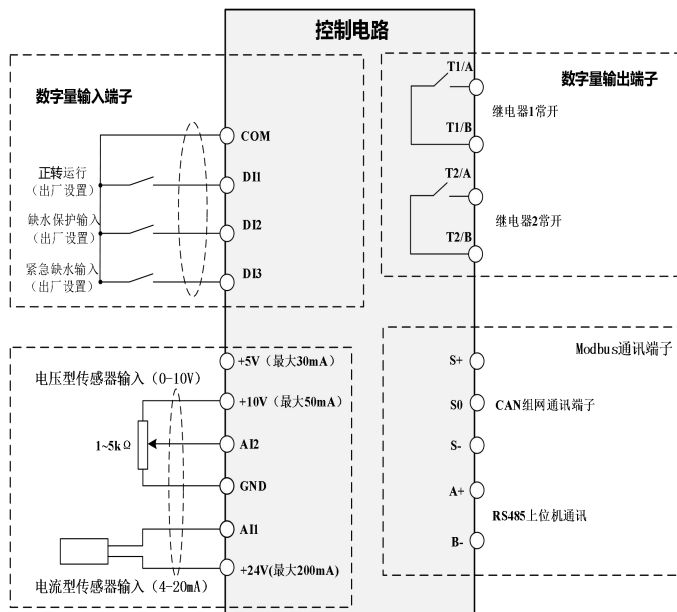
图 2-6-1 0.75kW-7.5kW 控制端子
