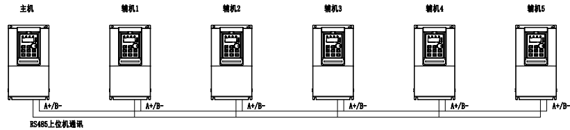
图 3-1-2 联机示意图
