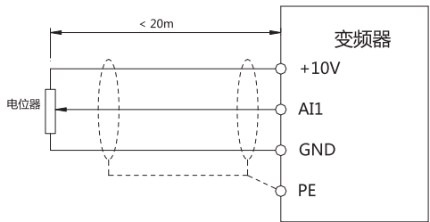
图3-16 模拟量输入端子接线示意图
