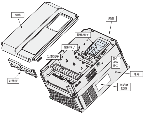
图2-2 变频器塑胶结构外型图
