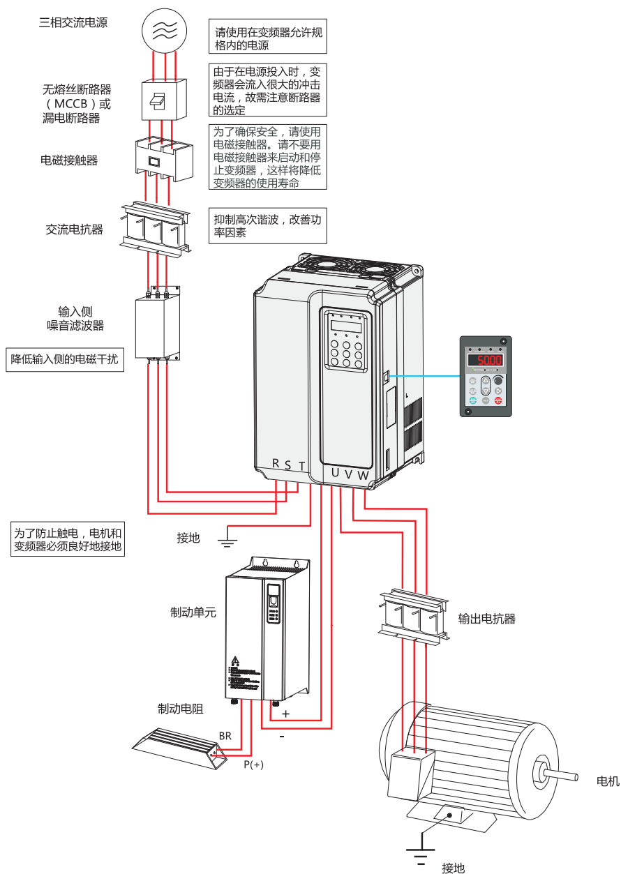
图2-4 系统构成图
