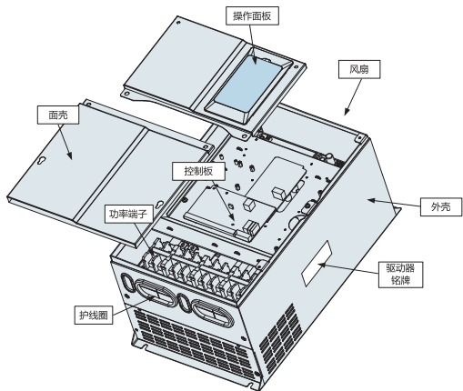
图2-3 变频器钣金结构外型图
