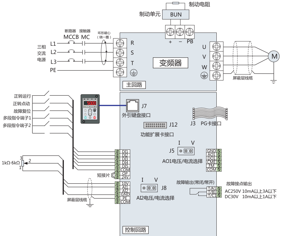
图3-22 变频器电气接线示例
