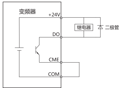
图3-21 数字输出端子接线示意图
