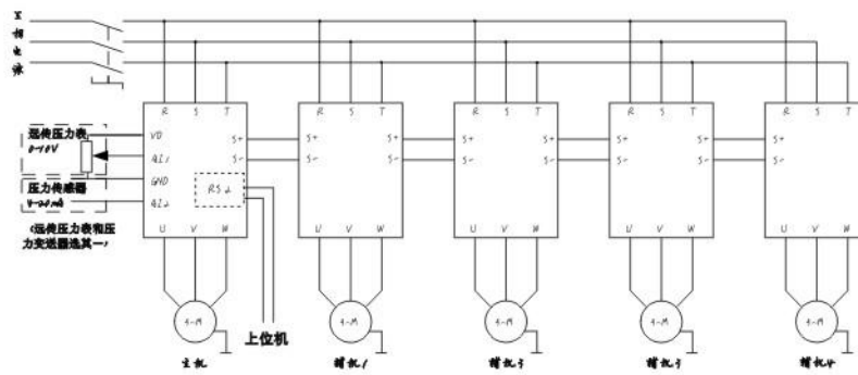
端子接线图（最多可控制5台辅机）
