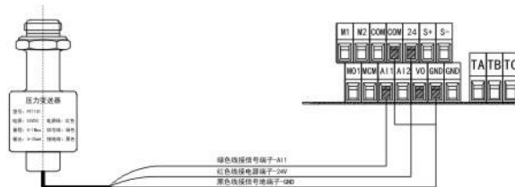
二线制压力变送器接线图
