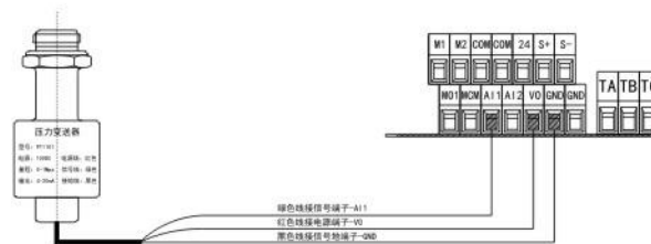
三线制压力变送器接图
